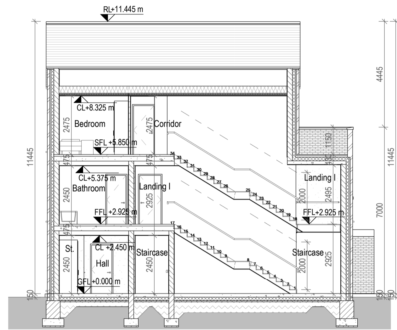
2 Section A-A 1:100
